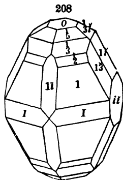
Sulphur.
